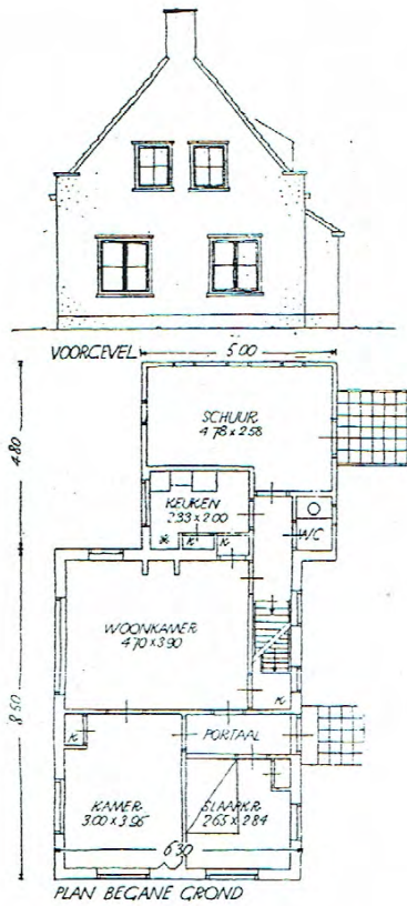
GRONINGEN. TYPE A3 KLAS.-INHOUD 303 M 3 ARCH.-BUR. VAN WIJK EN BROOS. GRONINGEN
