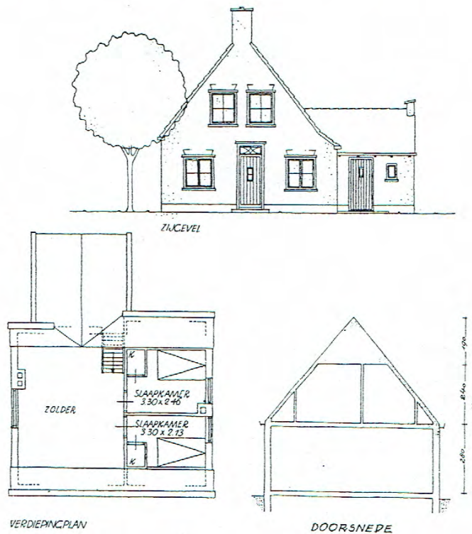
GRONINGEN. TYPE A4 KLAS.-INHOUD 277 M 3 ARCH.-BUR. VAN WIJK EN BROOS. GRONINGEN
