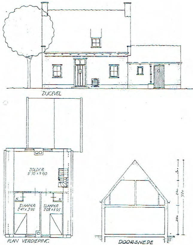
GRONINGEN. TYPE A3 KLAS.-INHOUD 303 M 3 ARCH.-BUR. VAN WIJK EN BROOS. GRONINGEN
