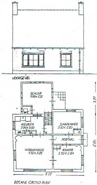
GRONINGEN. TYPE A4 KLAS.-INHOUD 277 M 3 ARCH.-BUR. VAN WIJK EN BROOS. GRONINGEN
