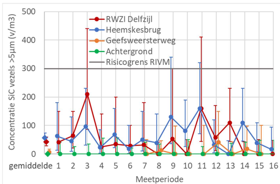
Figuur 1. Meetresultaten siliciumcarbide vezels op de drie hoofdmeetstations meetnet Oosterhorn in de periode 10 oktober 2018 tot en met 4 maart 2020 inclusief gewogen gemiddelde concentraties over de 16 meetperioden en vergelijking met de door het RIVM geadviseerde risicogrenswaarde van 300 vezels/m 3 (Advies 14725A01 – Afleiden indicatieve humane MTR-lucht voor siliciumcarbide-vezels, 1 april 2019)
