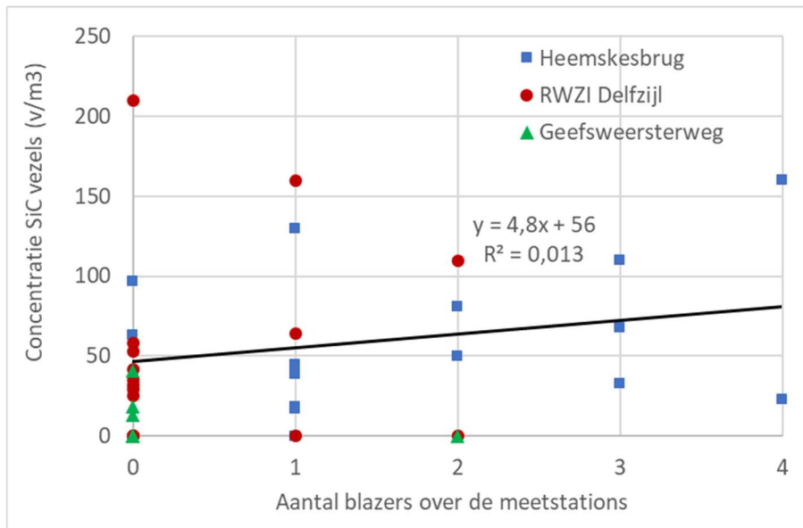
Figuur 2. De gemeten concentraties SiC vezels per meetperiode op RWZI Delfzijl, Heemskesbrug en Geefswesterweg uitgezet tegen het aantal opgetreden blazers dat over het betreffende meetstation is gegaan in dezelfde meetperiode.
