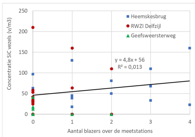
Figuur 3. De gemeten concentraties SiC vezels per meetperiode op RWZI Delfzijl, Heemskesbrug en Geefsweersterweg uitgezet tegen het aantal opgetreden blazers dat over het betreffende meetstation is gegaan in dezelfde meetperiode.
