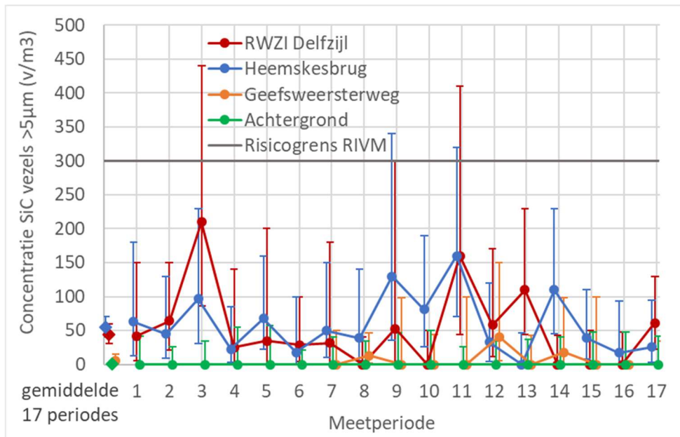
Figuur 2. Meetresultaten siliciumcarbide vezels op de drie hoofdmeetstations meetnet Oosterhorn in de periode 10 oktober 2018 tot en met 8 april 2020 inclusief gewogen gemiddelde concentraties over de 17 meetperiodes en vergelijking met de door het RIVM geadviseerde risicogrenswaarde van 300 vezels/m 3 (Advies 14725A01 – Afleiden indicatieve humane MTR-lucht voor siliciumcarbide-vezels, 1 april 2019)
