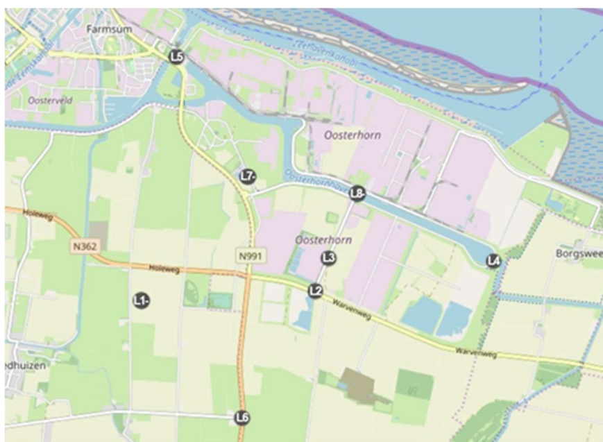
Figuur 1. Ligging van de huidige meetstations van het meetnet in de omgeving van industriegebied Oosterhorn (de meetstations in de woonkernen Borgsweer en Wagenborggen staan niet ingetekend in de figuur).
