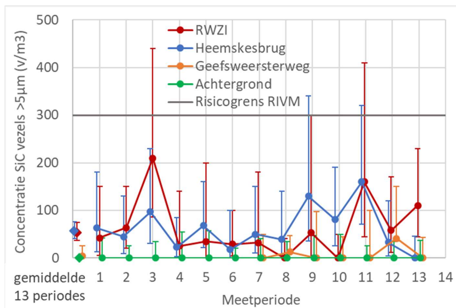
Figuur 1. Meetresultaten siliciumcarbide vezels op de drie hoofdmeetstations meetnet Oosterhorn in de periode 10 oktober 2018 tot en met 4 december 2019 inclusief gewogen gemiddelde concentraties over de 13 meetperioden en vergelijking met de door het RIVM geadviseerde risicogrenswaarde van 300 vezels/m 3 (Advies 14725A01 – Afleiden indicatieve humane MTR-lucht voor siliciumcarbide-vezels, 1 april 2019)
