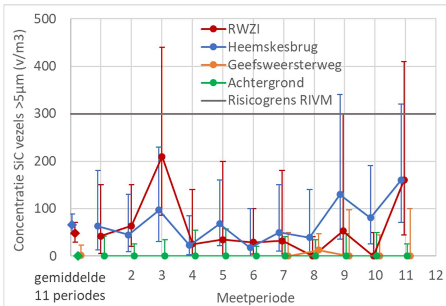
Figuur 1. Meetresultaten siliciumcarbide vezels op de drie hoofdmeetstations meetnet Oosterhorn in de periode 10 oktober 2018 tot en met 1 oktober 2019 inclusief gewogen gemiddelde concentraties over de 11 meetperioden en vergelijking met de door het RIVM geadviseerde risicogrenswaarde van 300 vezels/m 3 (Advies 14725A01 – Afleiden indicatieve humane MTR-lucht voor siliciumcarbide-vezels, 1 april 2019)
