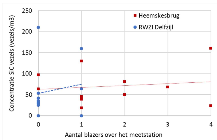
Figuur 2. De gemeten concentraties SiC vezels per meetperiode op RWZI Delfzijl en Heemskesbrug uitgezet tegen het aantal opgetreden blazers dat over het betreffende meetstation is gegaan in dezelfde meetperiode.
