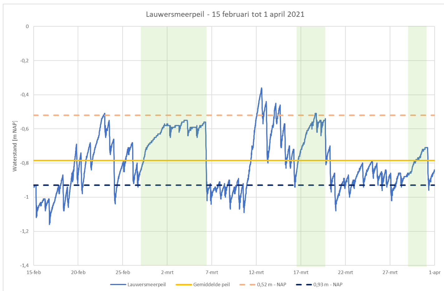
Figuur 1.1: Daggemiddelde oppervlaktewaterstand Lauwermeer 15 febr. - 1 april 2021. In de groene periodes is de waterstand van het Lauwersmeer actief verhoogd
