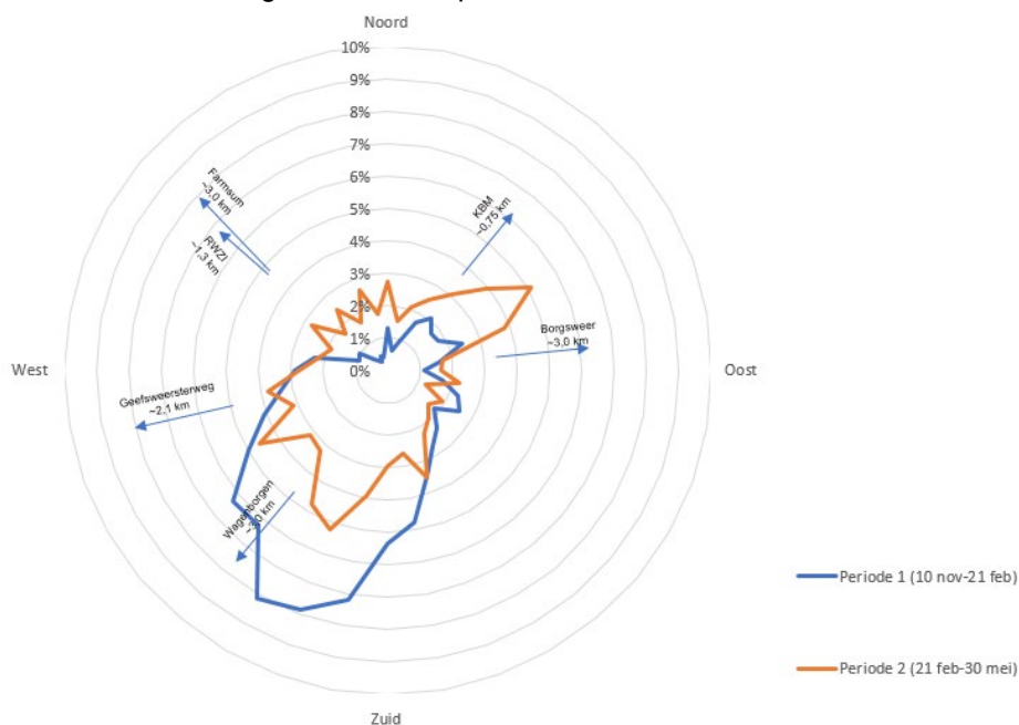
Figuur 2. Windroos met uurgemiddelde windrichtingen tijdens de meetperioden van het nieuwe meetnet Oosterhorn 2023 (10 november 2021 tot en met 30 mei 2023).
