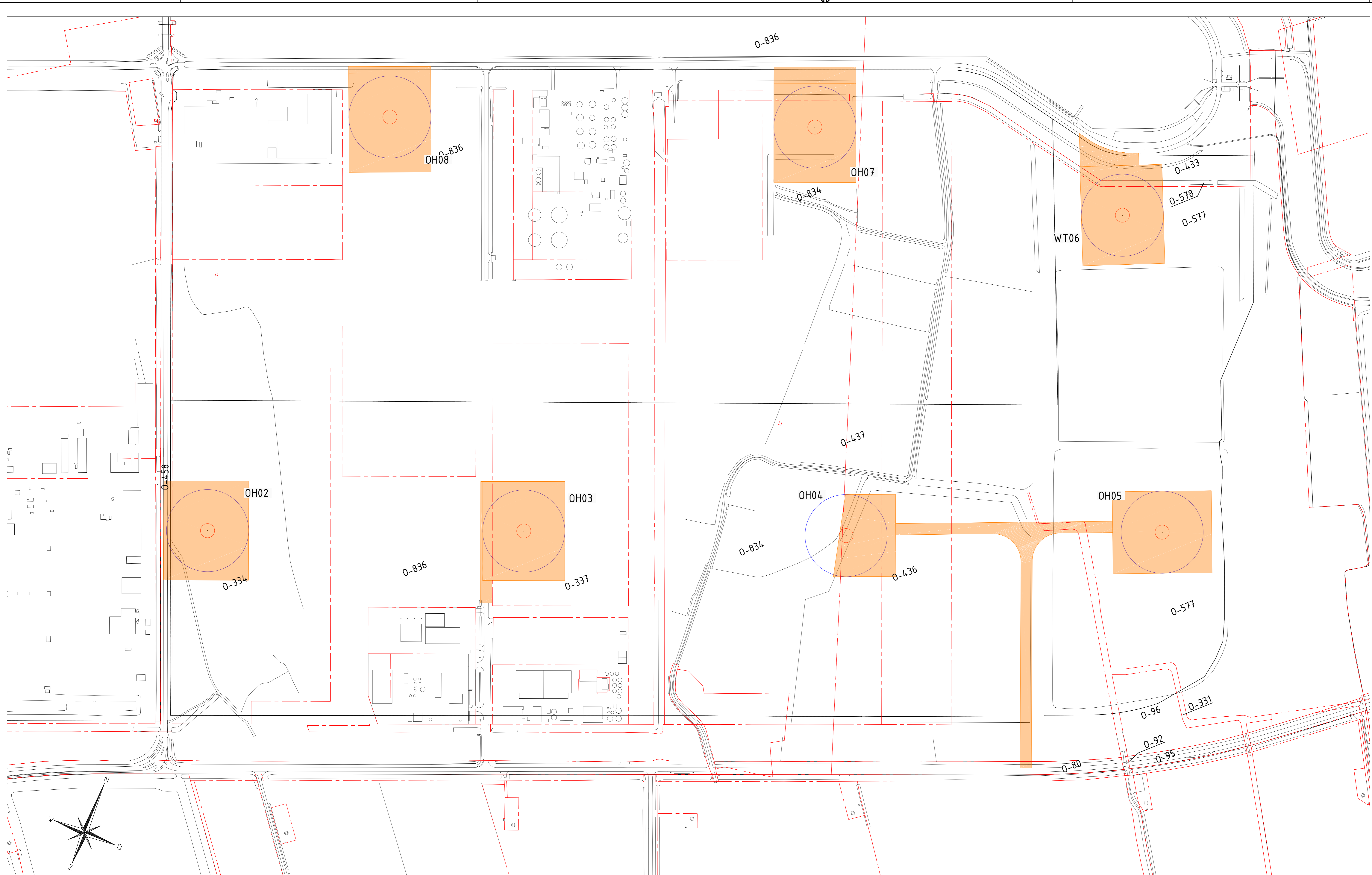
Inrichtingsplan Oosterhoorn OH02 t/m OH08
